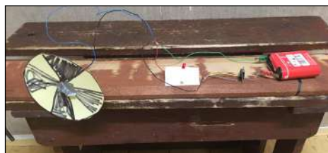
Vysílačka skupiny Silver A
