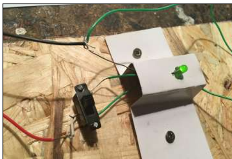
Spínač a dioda
