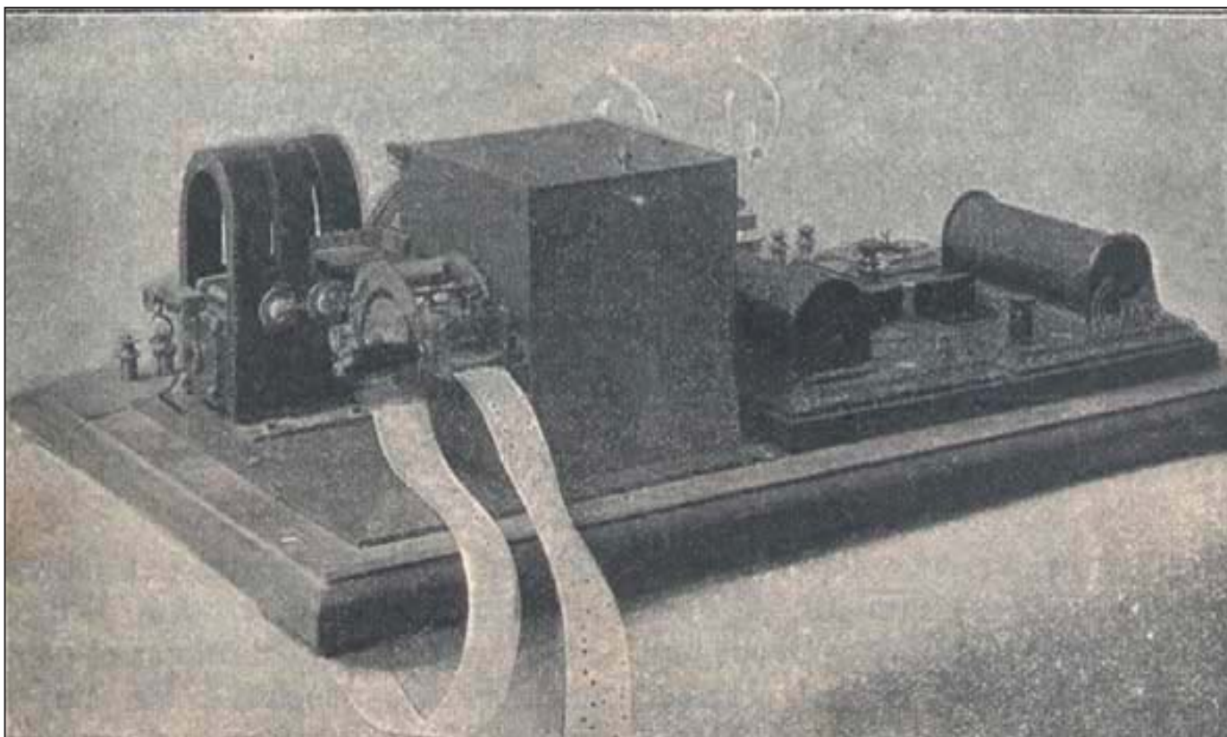
Odesílací přístroj rychlotelegrafu Virágova.
