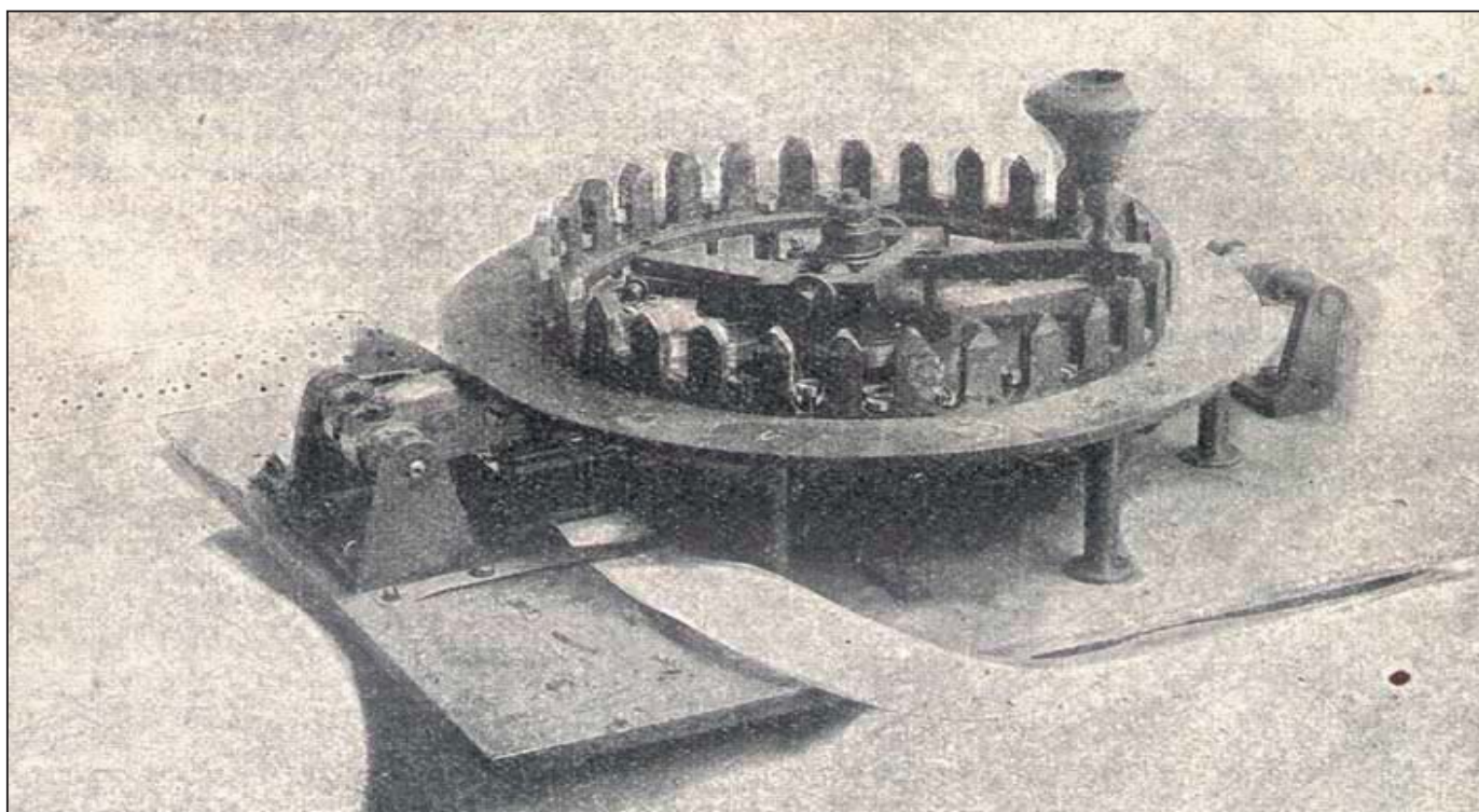
Perforátor pro rychlostní telegraf Viragův
